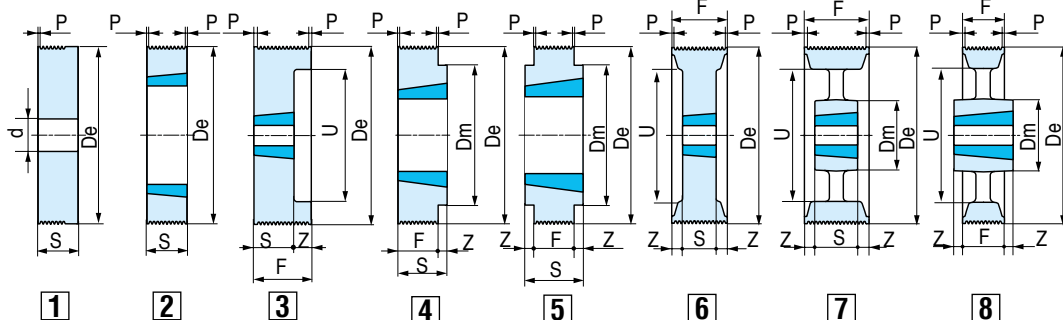
POULIES PPL à moyeu amovible PPL MA x D x nb gorges G
